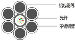
束管式结构图
