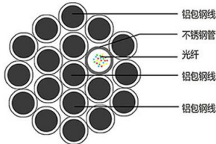
层绞式结构图
