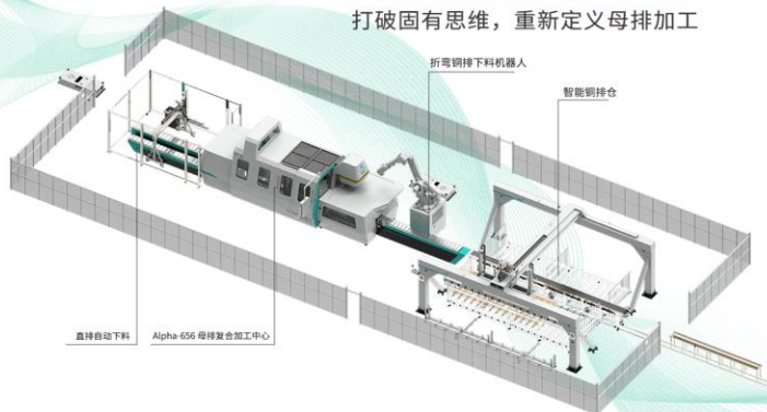
Alpha-656 母排智能加工系统
