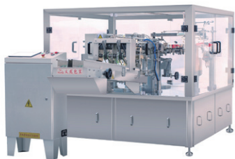
YL-双列给袋式包装机
