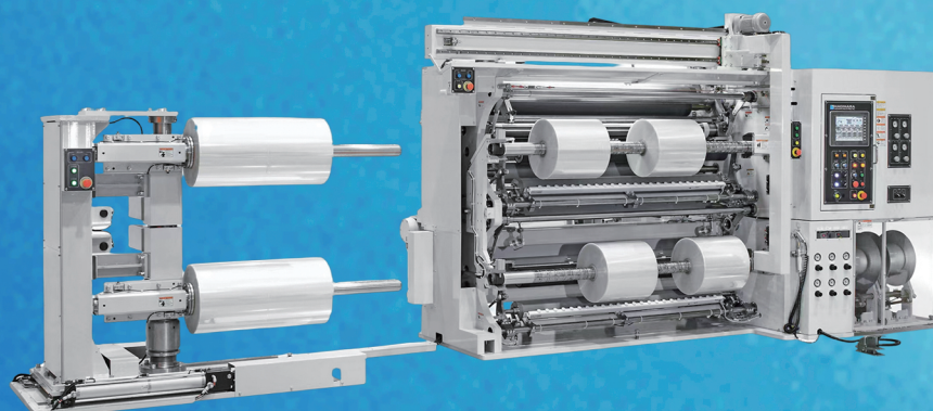
HDF-306V-1300 上下 2 轴中心驱动分切机
