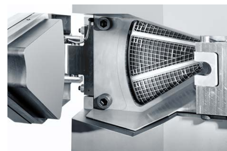
RSFgenius 旋转过滤系统兼具工艺稳定、压力恒定的优势，且集成了自清洁功能。（过滤网细节图）
