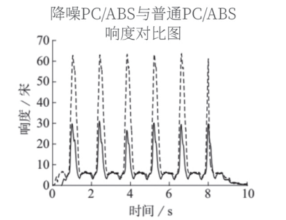
兆维科技降噪PC/ABS材料在同等测试条件下响度明显且恒定的低于普通PC/ABS。
