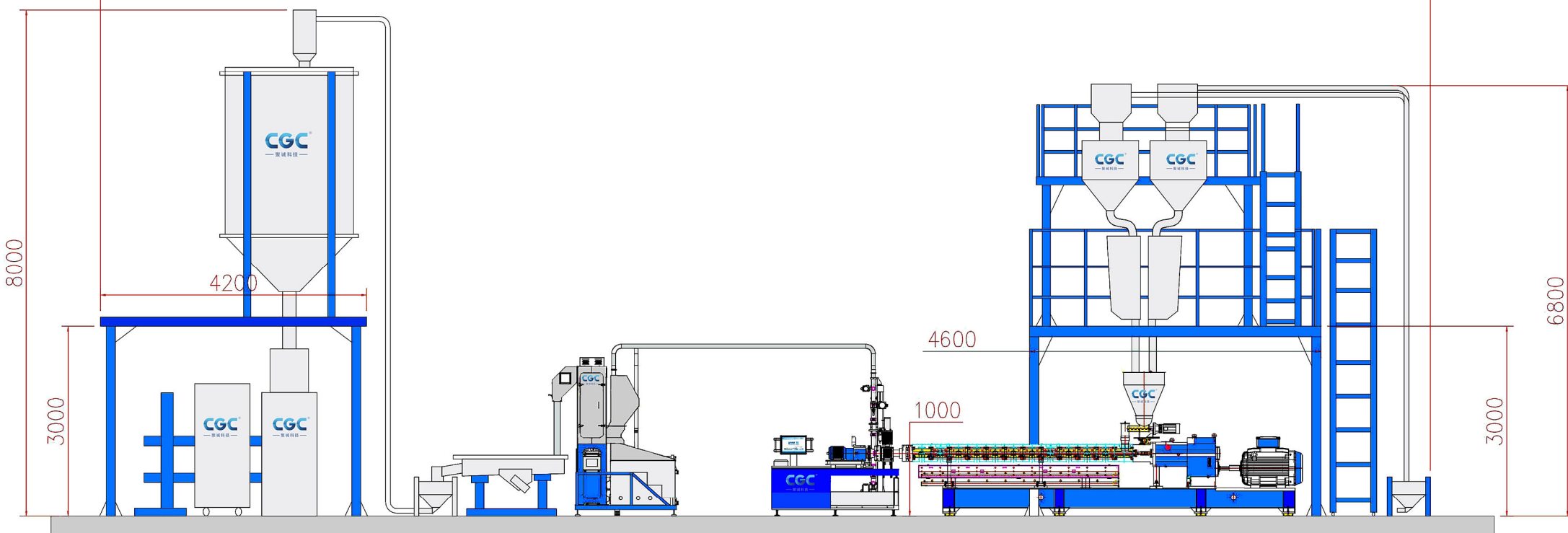
UWP®品牌水下造粒生产配置A: 混料-喂料-挤出机-换网器 (熔体泵) -开车阀-切粒机-水系统-离心脱水机-出料-干燥-包装
